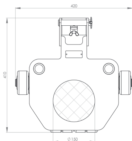
JLF 3,5 | Art.No. 16 035 085-D | Draufsicht | Top view
