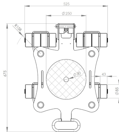
JKB 6 K | Art-No. 14 061 085-P | Draufsicht | Top view
